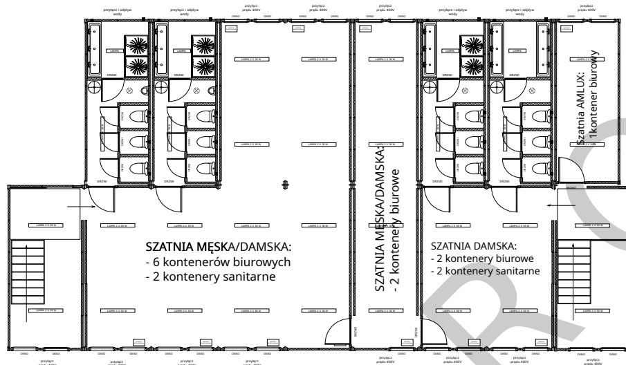
I PIĘTRO
